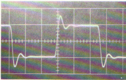
Stabilité inconditionnelle sur charge semi-capacitive.
