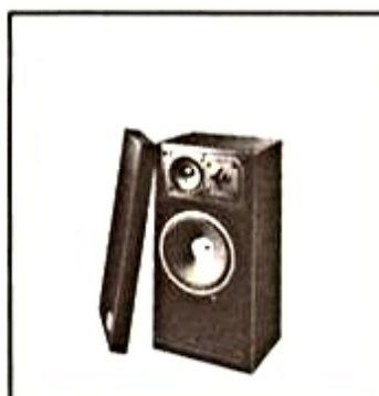
3a - 340. Très haute fidélité. 3 voies bibliothèque. HP basse à grande excursion et haute énergie. HP aigu à dôme à ferrofluide. HP médium à cône clos. Mise en phase optimale des HP basse et médium.
