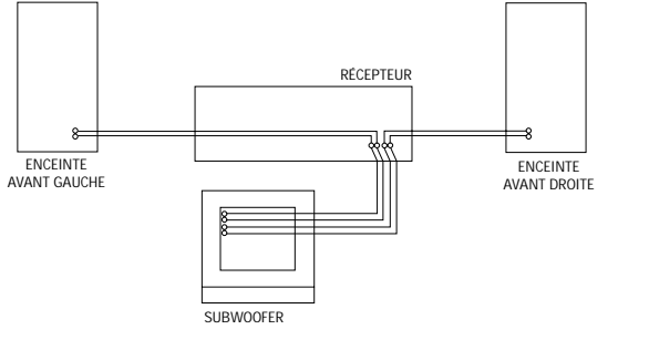
Raccordez les fils de enceinte des sorties sur le récepteur avant gauche et droite à bornes IN de subwoofer gauche et droite, et les enceintes avants gauche et droite
