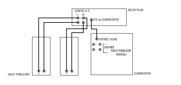
Connecter un câble audio entre la Sortie de Subwoofer ou la Sortie LFE (Canal Effets Basse Fréquence) sur l'arrière de votre Récepteur et le jack d'Entrée Ligne sur l'arrière du subwoofer.
