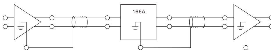
Abb. 4: Signalfuß (symmetrische Beschaltung)
