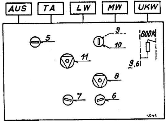
Spulensatz von unten gesehen
