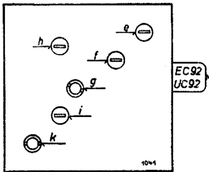
Spulenplatte von oben gesehen
