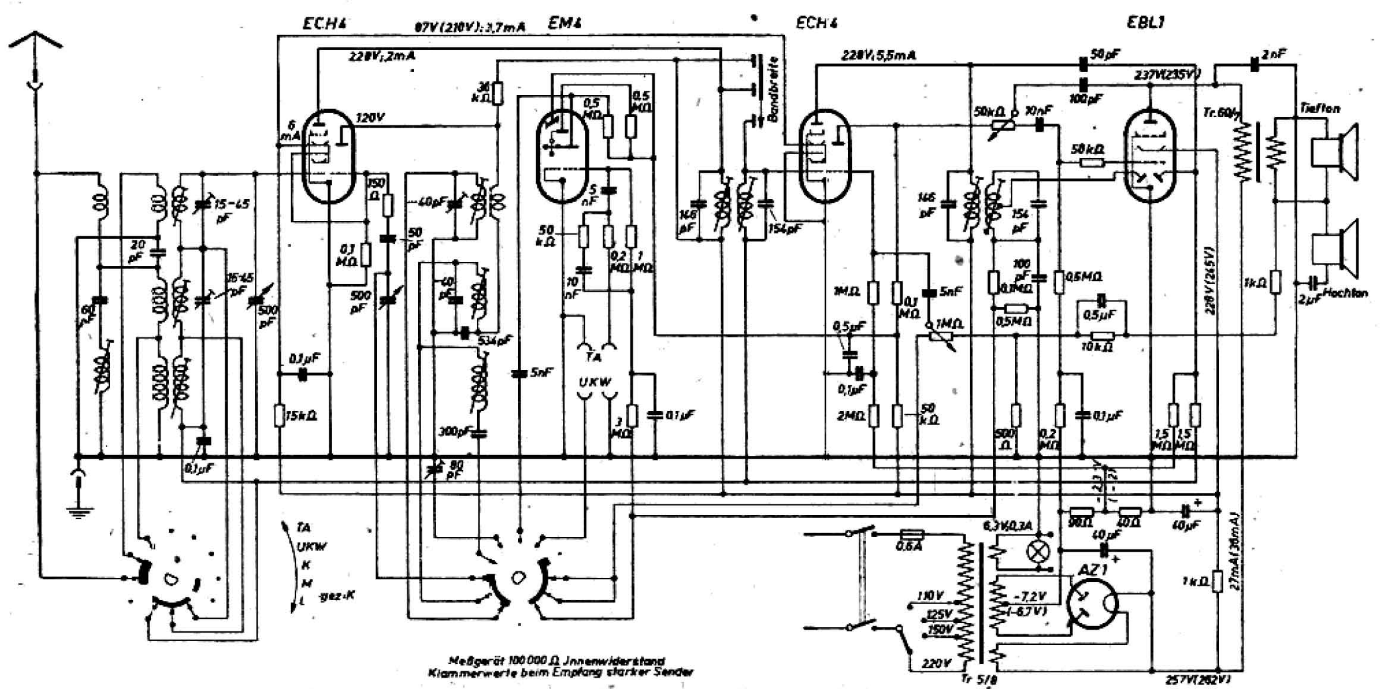
Grundig „Musikschrank I“ 988 W
