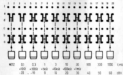
Miniatürkstenschalter (Bestückungsseite) MINIATURE KEY-SWITCH (COMPONENT SIDE) 40102-030.00
