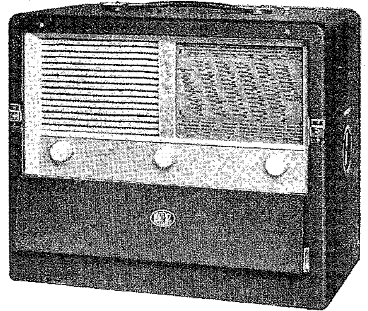
Das Aeussere des 5-Röhren-6-Kreis-Super mit eingebauter Rahmenantenne. Wellenbereiche 16,5—50 m, 185—580 m, 725 bis 2100 m.
