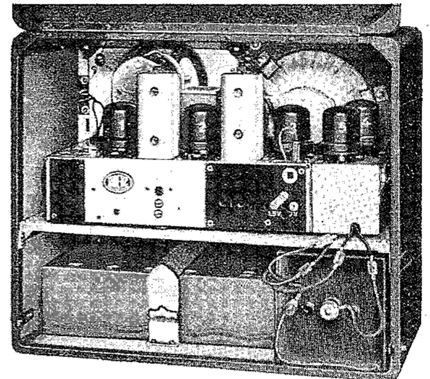
Rückansicht des Koffers bei abgenommener Rückwand
