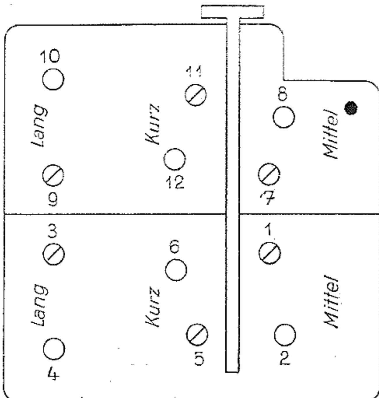
Chassis unten
