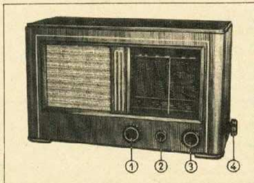
① Lautstärkereglер mit Netzschalter, ② Klangfarbenregler, ③ Abstimmung, ④ Wellenbereichshalter
