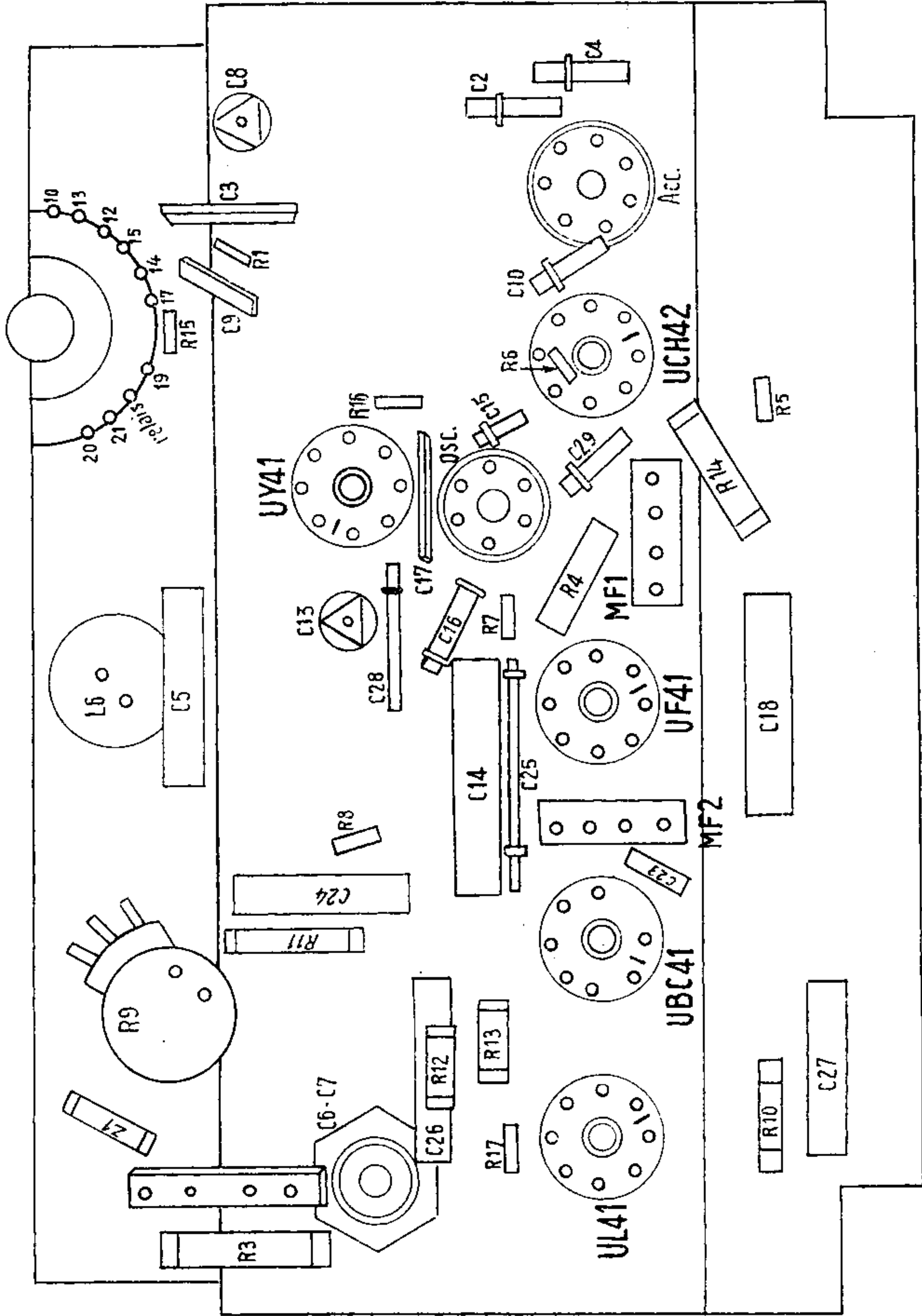
Disposition des résistances et des condensateurs à l'intérieur du châssis des récepteurs BF111U et RA15U.
