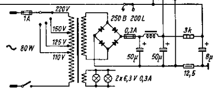
AM/FM-Großsuper (1952) mit multiplikativer Mischstufe ECH 42 bei AM und FM, HF-Vorröhre EF 85, zweistufiger ZF-Verstärkung und Radiodetektor (Telefunken Opus).
