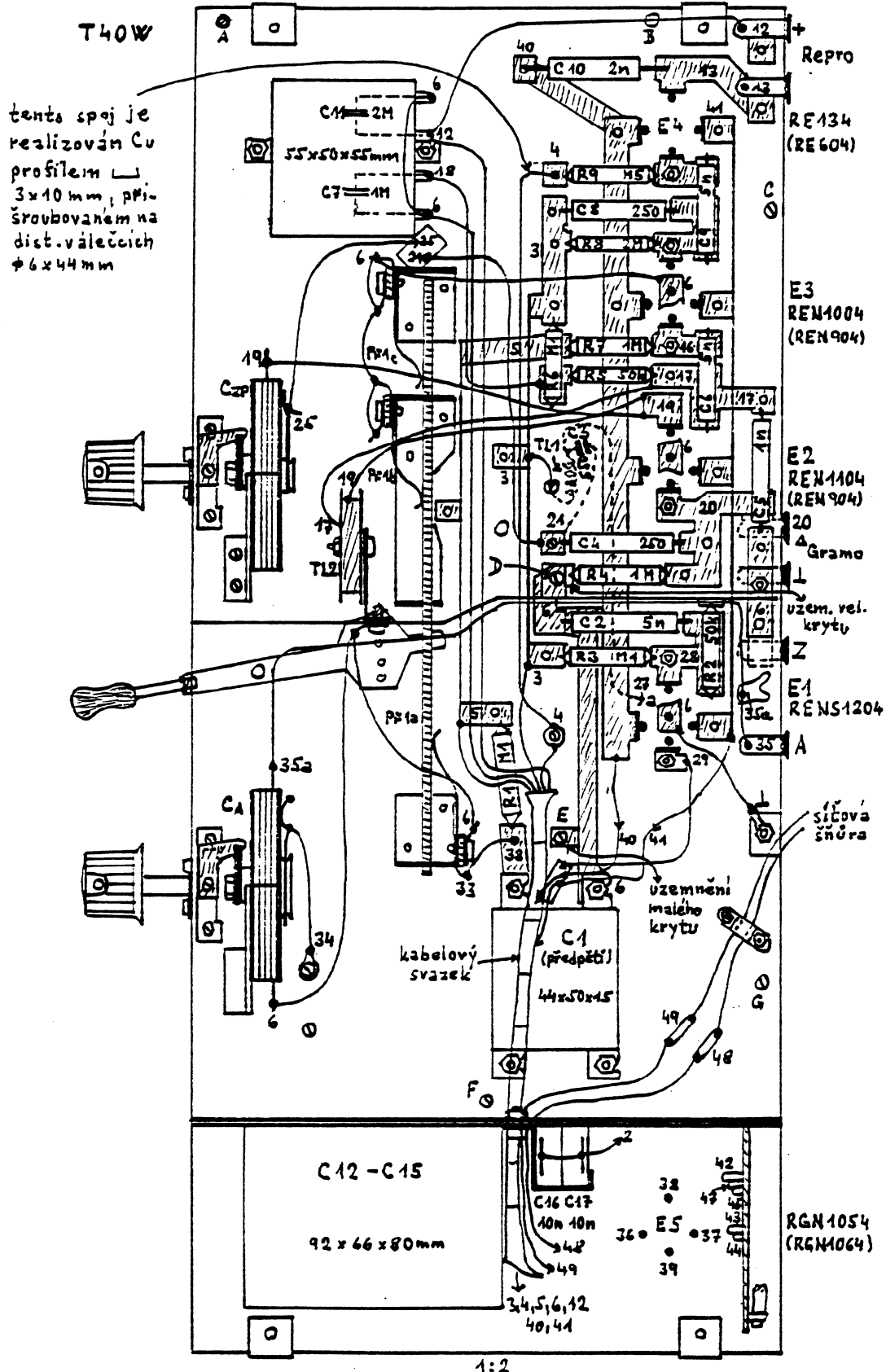
Obr. 2. Zapojovací plánek (pod šasi).
