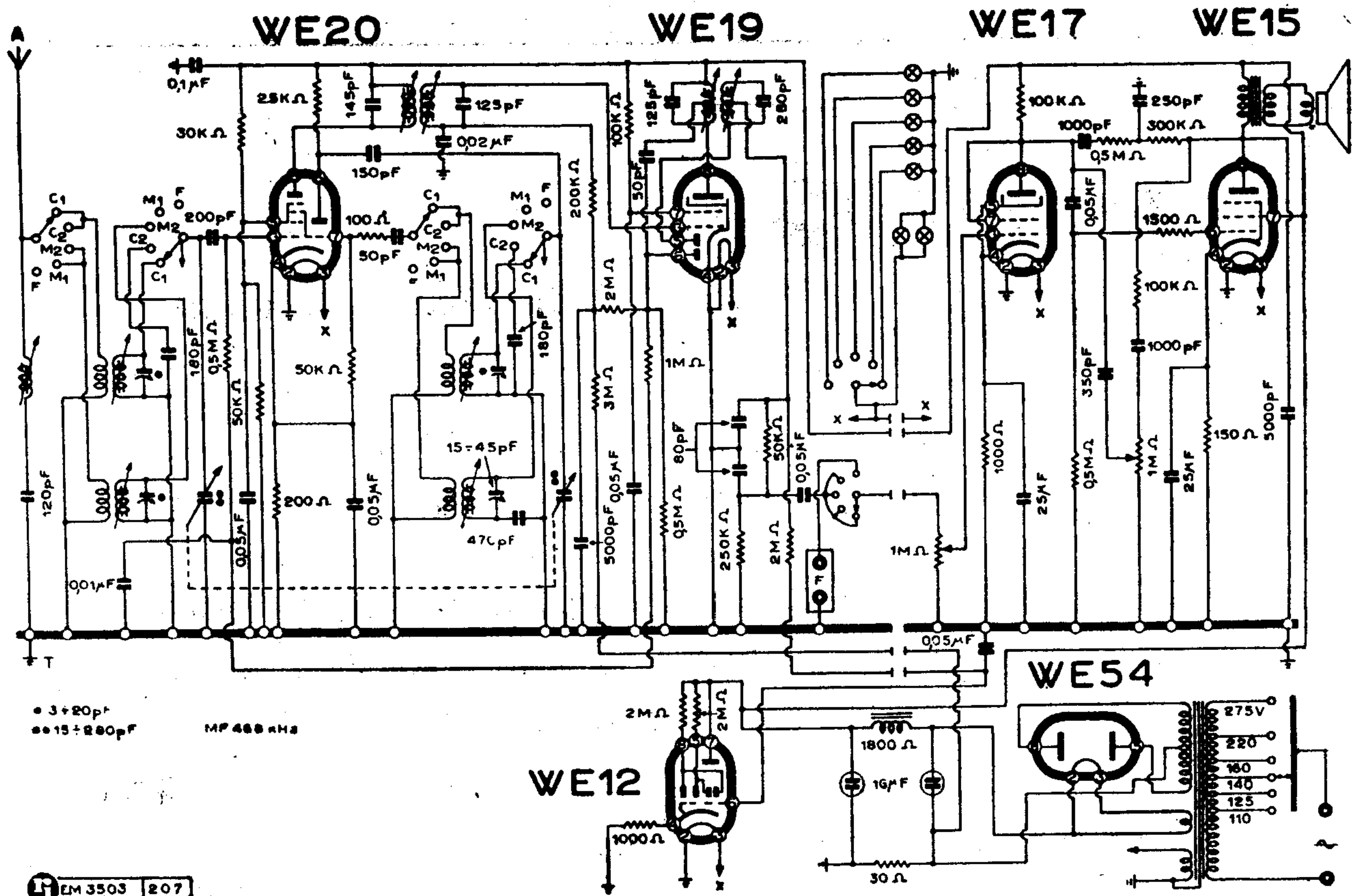
COMP. RADIORIC. TELEFUNKEN - MOD. « T 6 »
